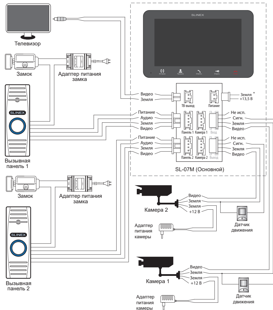
Схема 1. Подключение вызывных панелей, камер и телевизора к домофону SM-07M.
