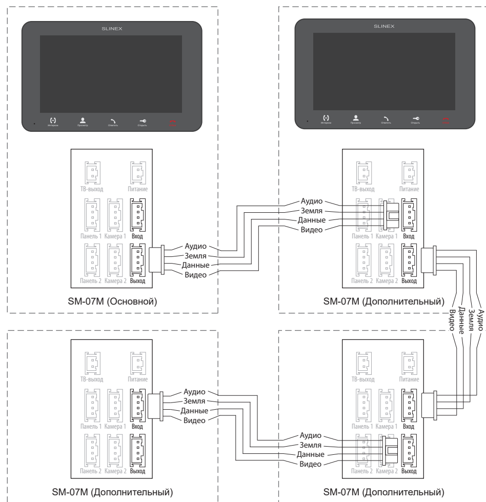
Схема 2. Подключение системы домофонов SM-07M.
