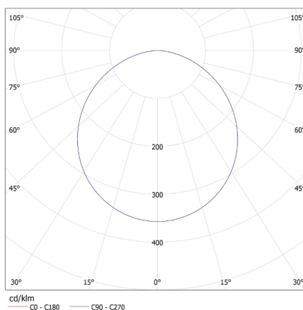
MILED (kat 31083) SP LED N 18W NW-R / LDC (Polar)
