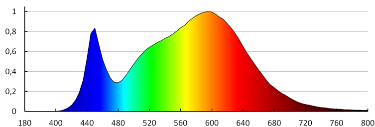
MILED (kat 31083) SP LED N 18W NW-R / LDC (Polar)
