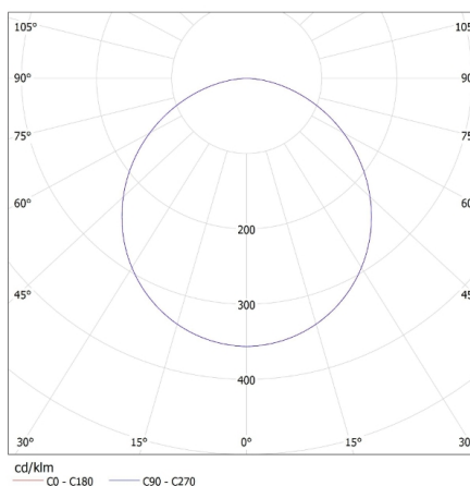
MILED o (kat 31082) SP LED N 18W NW-S / LDC (Polar)
