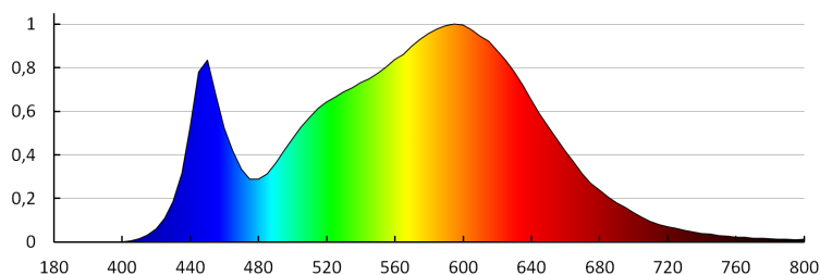
MILED o (kat 31082) SP LED N 18W NW-S / LDC (Polar)
