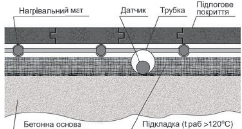
Розріз підлоги мат EASYTHERM EMF
