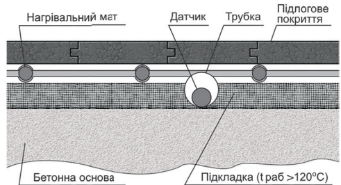
Розріз підлоги мат EASYTHERM EMF
