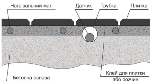
Розріз підлоги мат EASYTHERM EM
