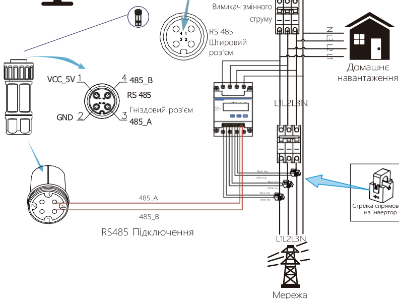
Малюнок 7.12 Схема підключення лічильника CHNT
