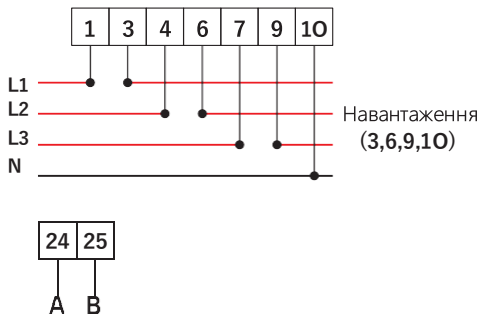
Малюнок 7.28 Лічильник CHNT
