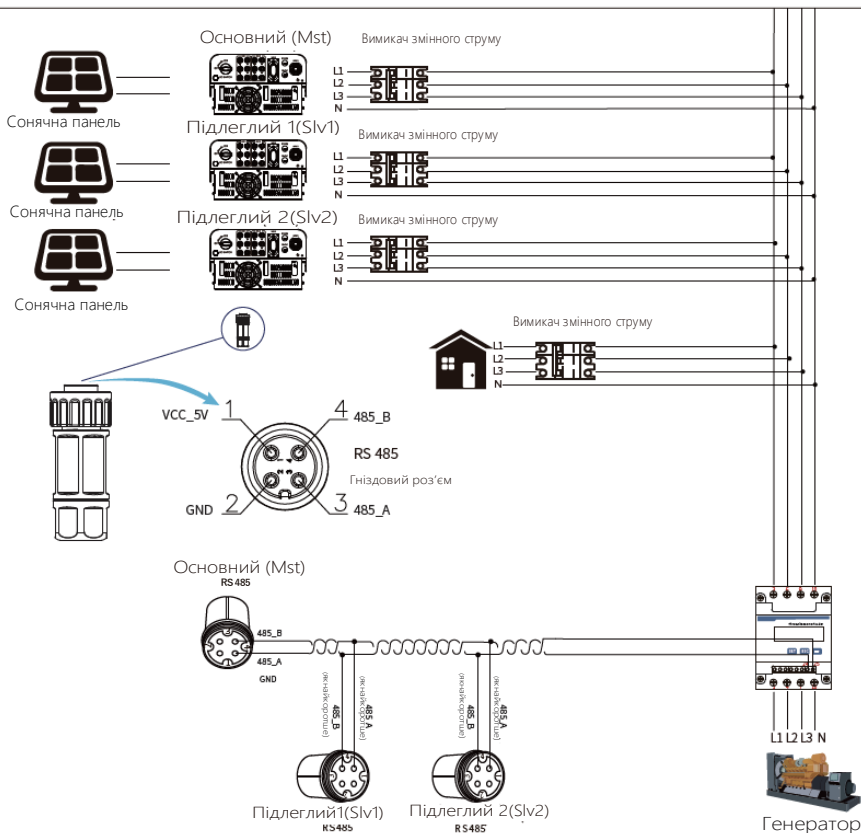
Малюнок 7.29 Схема підключення СНТ (Прохідна схема)
