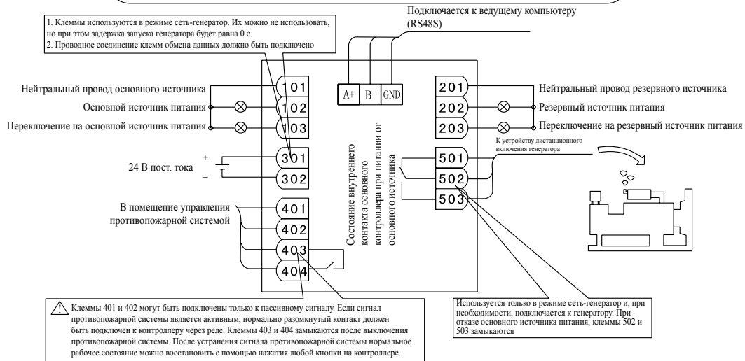
Типовое применение
