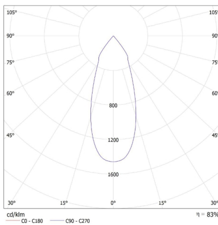
KANLUX S.A. (kat 22844) HIMA LED 33W-NW-B / LDC (Polar)
